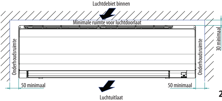
Vereiste ruimte voor service en ventilatie
