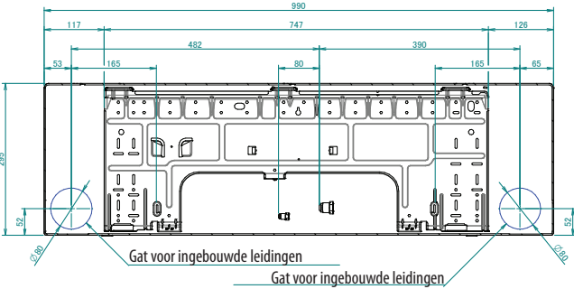
Standaardlocatie van gaten in de wand
