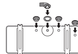
Tapón de desagüe
