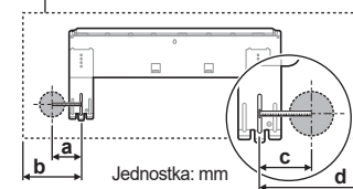
Rama jednostki wewnętrznej
