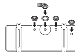
Verschlussstopfen
